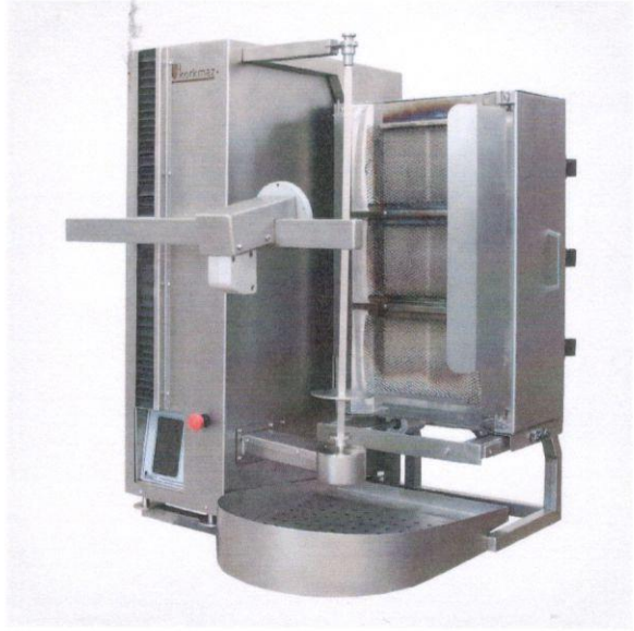
1.2 Otomatik Döner Pişirme, Kesme, Dilimleme Ve Tartma Makinası
